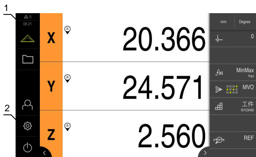
图 4: 用户界面
